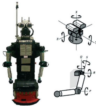
図 4.1: Robovie II の駆動機構
